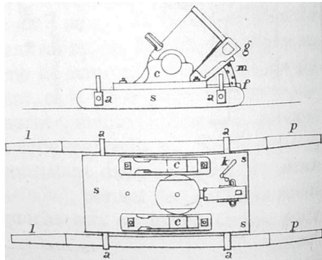
Fig. 2 : Mortier de 15 cm. Affût et profil de la pièce.
