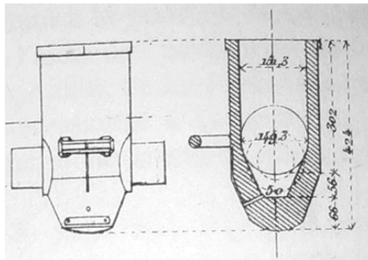
Fig. 1 : Mortier de 15 cm. Canon.
